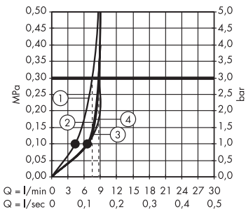
Croma 100 Vario 28537000
