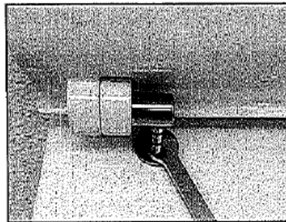
07 Stringere con la chiave in dotazione il fissaggio. Tighten the fixing screw by using the provided key.
